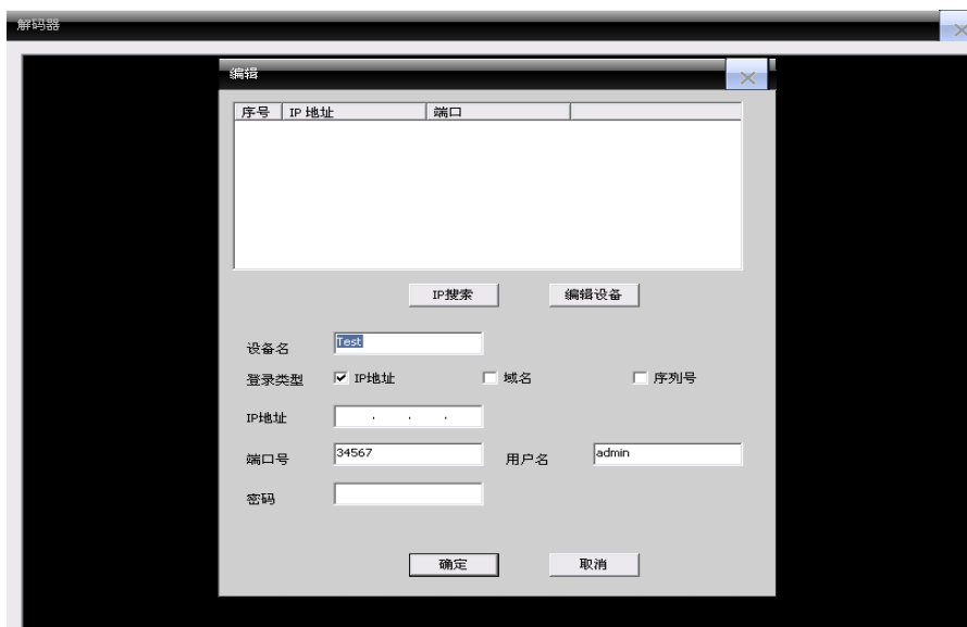
图 39 添加解码器
