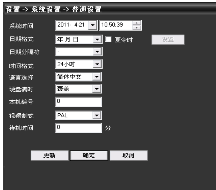
图 16 普通设置
