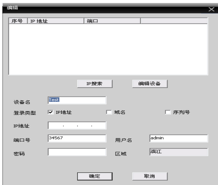
图 3 添加设备
