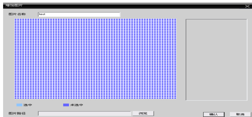
图 45 选择图片
