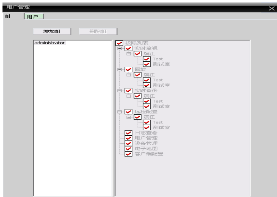
图 30 组管理
