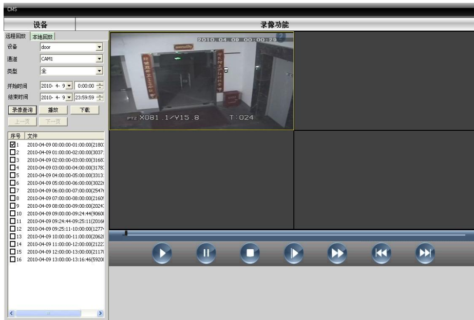
图 32 回放界面
