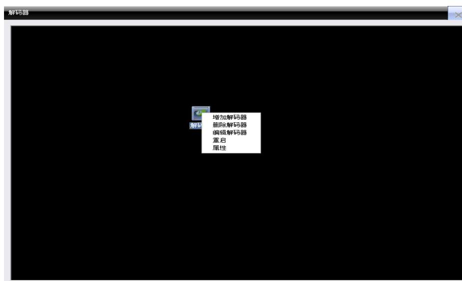
图 40 配置解码器
