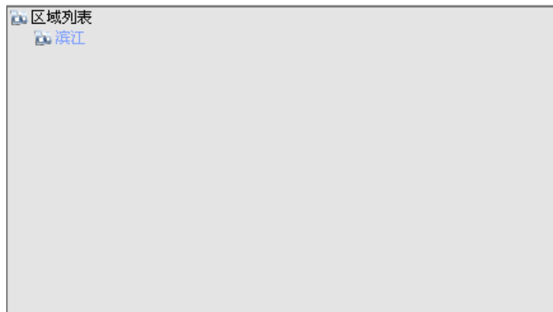
图 2 添加区域
