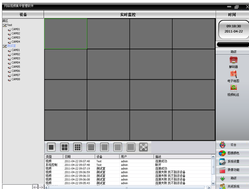
图 37 高级
