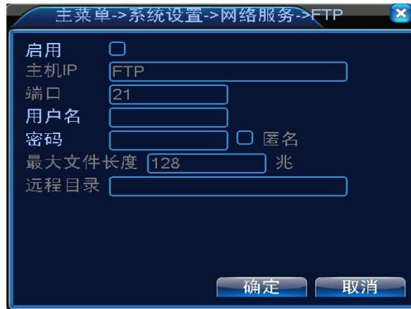
图 4.22 FTP 设置
