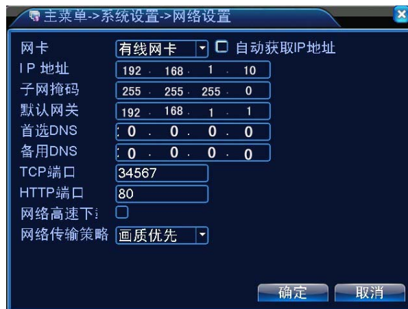
图 4.15 网络设置
